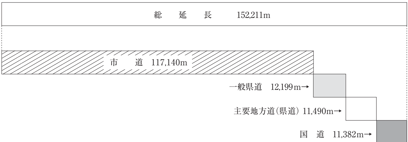
消雪パイプ敷設状況(令和3年3月31日現在) [8-3参照]
