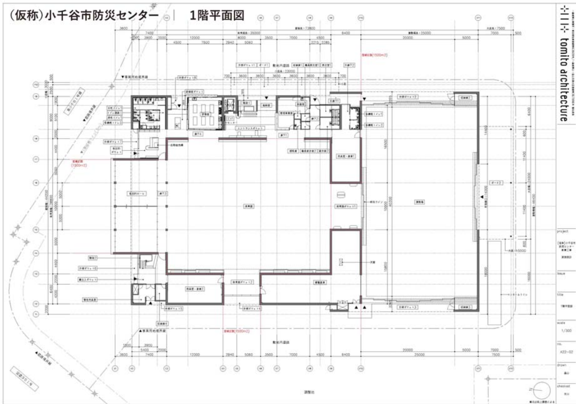
(仮称)小千谷市防災センター 図面
